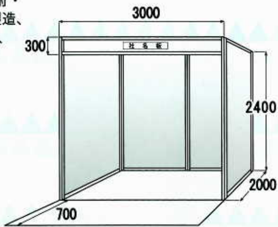
小間仕様 単位:mm
